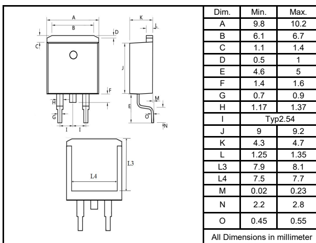
T0-263C
